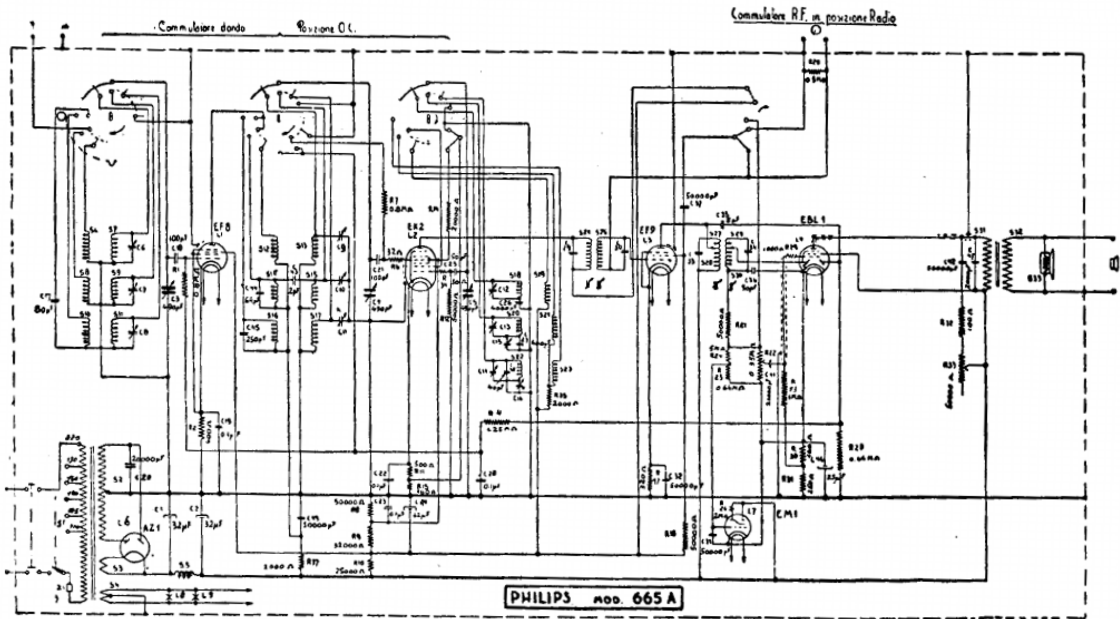
PHILIPS RADIO — Mod. 665 A — Produzione 1938-39. — Gamme: c. (18-5)), m. (210-575), l (200-2000). Media frequenza: 468 kHz.
